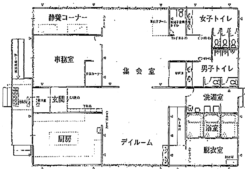
図：サポートセンター千歳平面図
